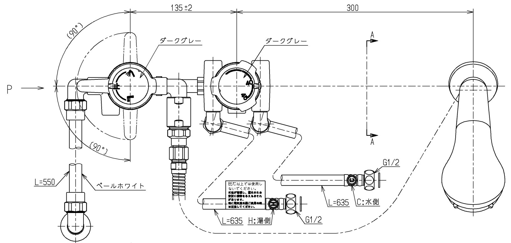
水栓取付け位置(フリー)
